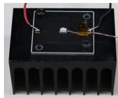
写真5 フィン下向き 空気の流れを妨げた向き)
