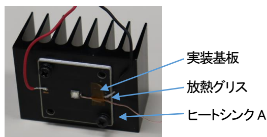
写真2 評価した光源の構成
