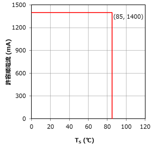
図1 T_S - 許容順電流特性
