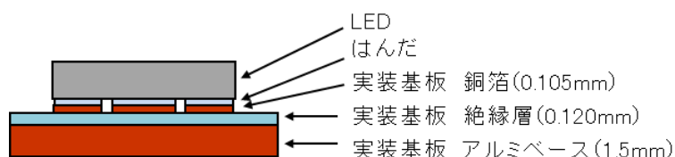
図3 実装構造
