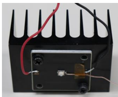
写真4 フィン垂直 (弊社設置向き)
