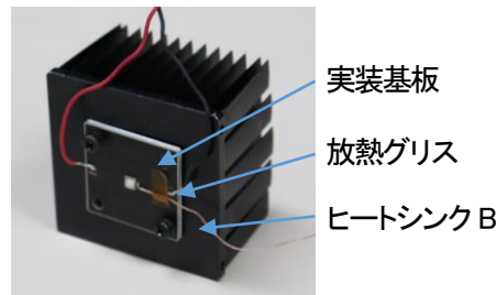
写真3 評価した光源の構成
